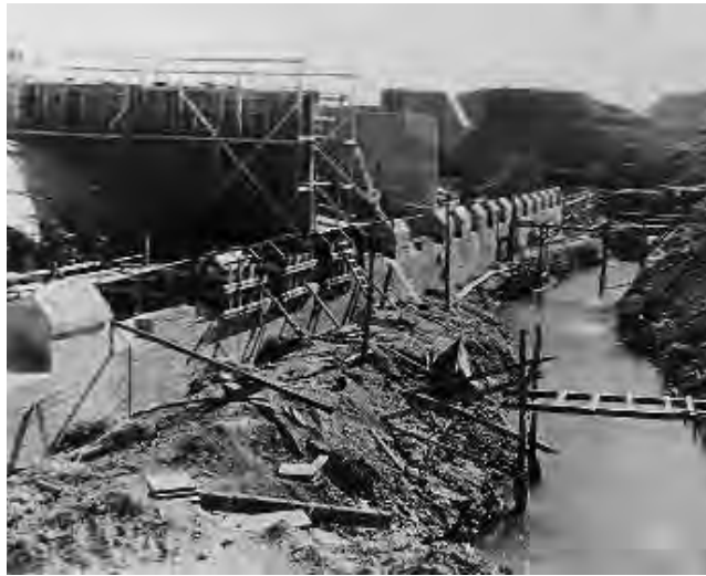
El puente - dique se terminó de construir en 1972. Esta foto pertenece a una etapa de su construcción en 1966.
